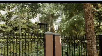
CodeX
